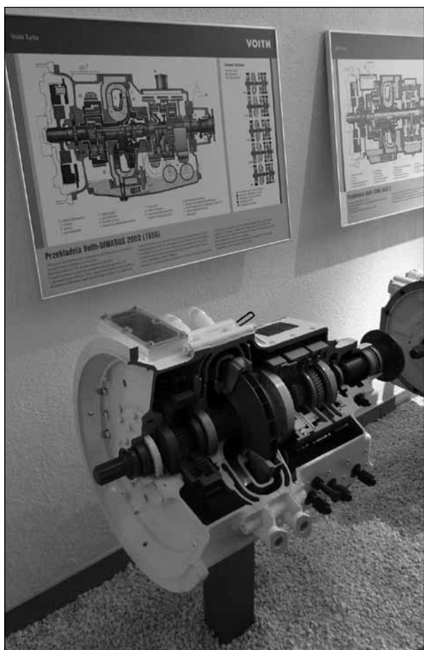
Eksponat z przekrojem automatycznej przekładni autobusowej
