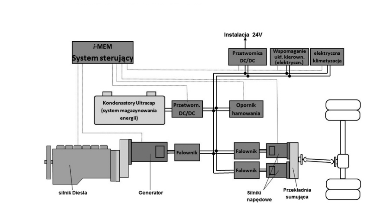
Rysunek 1 - Schemat hybrydowego układu napędowego
